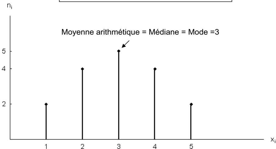
Figure 6 : Distribution parfaitement symétrique
