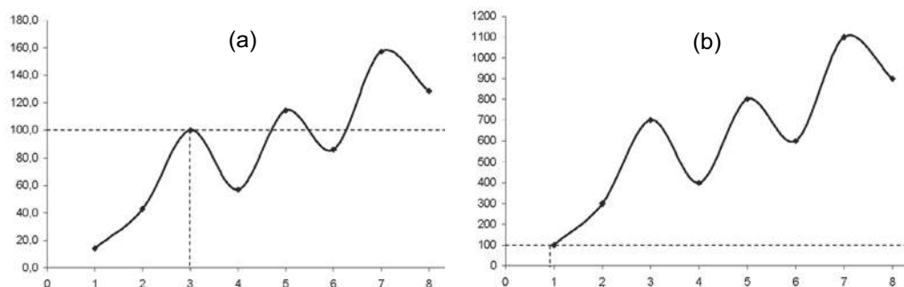
Figure 1 : Représentation graphique d'une série indice
