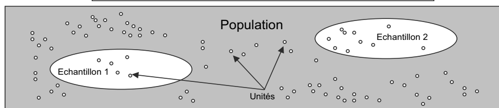
Schéma 2 : Unités statistiques, population, échantillons
