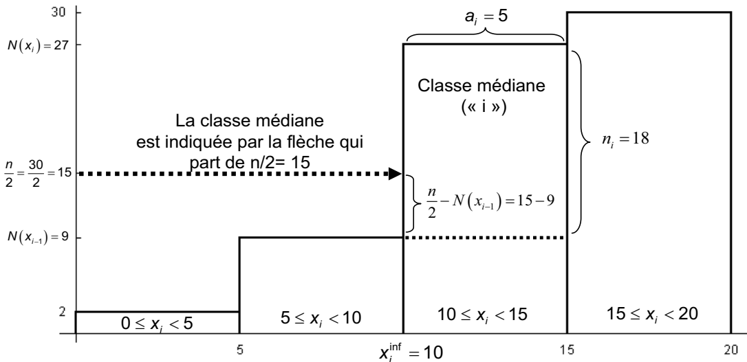
Figure 2 : Histogramme des effectifs cumulés
