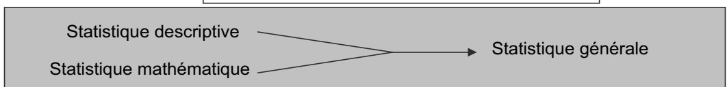
Schéma 1 : Les deux branches de la statistique
