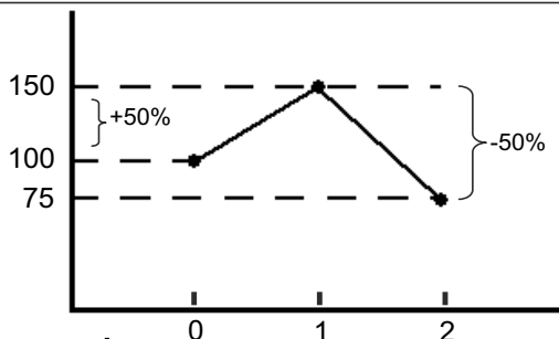
Figure 1 : Une hausse de 50% suivie d'une baisse de 50%
