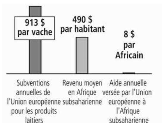
Figure 14 : Un beau graphique vaut mieux qu'un long discours
