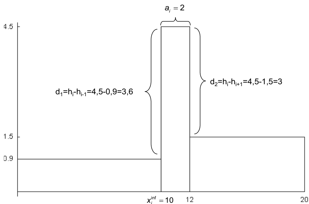
Figure 5: Calcul du mode quand les classes sont d'inégales amplitudes
