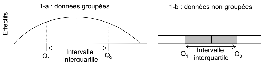
Figure 1 : La notion d'intervalle interquartile
