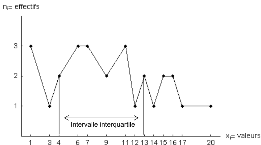
Figure 4 : L'intervalle interquartile, données groupées
