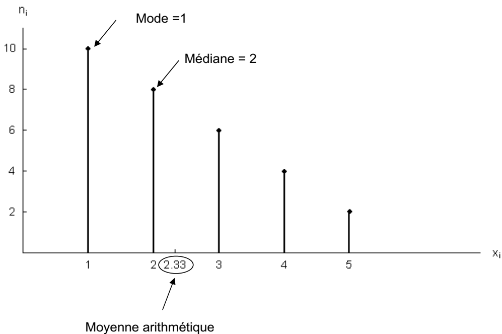
Figure 7 : Distribution étalée à droite
